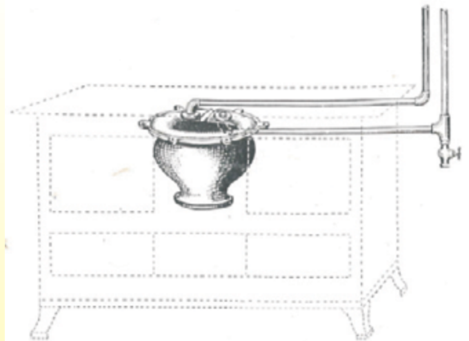
Intercambiador de calor "Bouilleur" montado en el interior de una estufa (Catálogo de Ets Demoulin, Farcennes, 1932, Ultimheat Museum)
